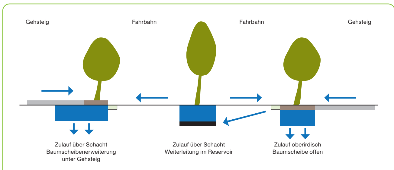
Darstellung einiger Regenwasserversickerungsmöglichkeiten in bzw. über Baumscheiben entlang von Straßen
